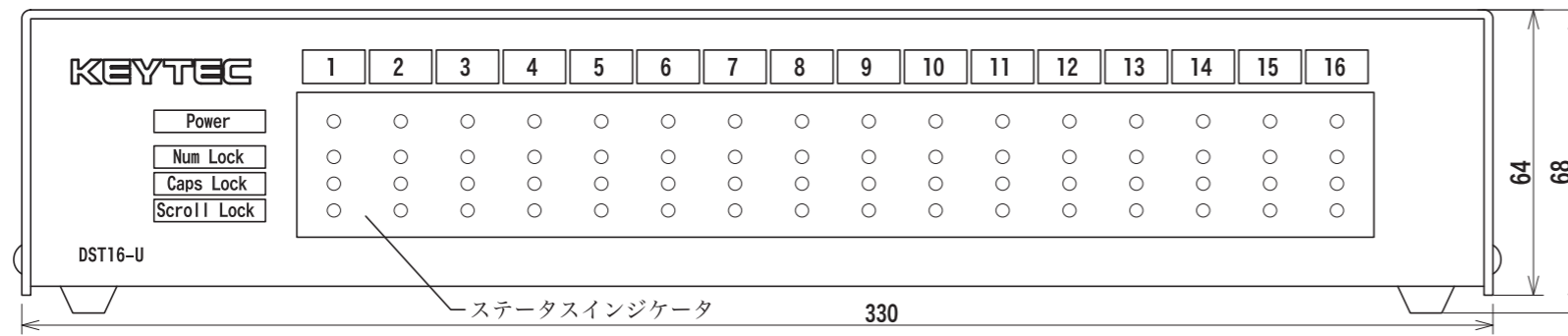
正面図
