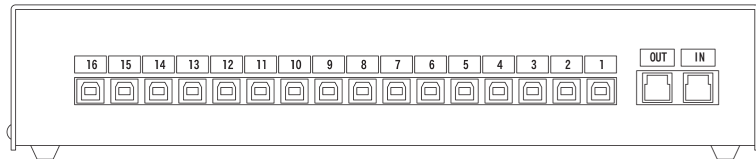
背面図
